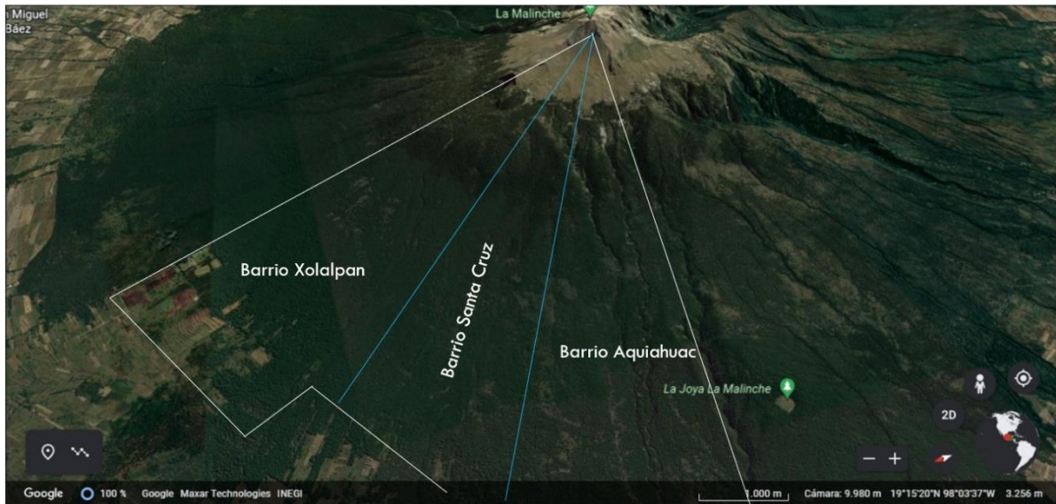
Mapa 2. Muestra de la extensión territorial boscosa que corresponde a San Francisco Tetlanohcan. La imagen satelital fue obtenida de Google maps y el trazo aproximado fue hecho a partir de información recabada por propietarios de los tres barrios. Realizado en enero de 2022.
